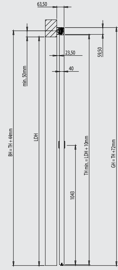
ZEICHNUNG PLANE0 60, FÜR HOLZTÜREN DRAWING PLANE0 60, FOR WOODEN-DOORS
