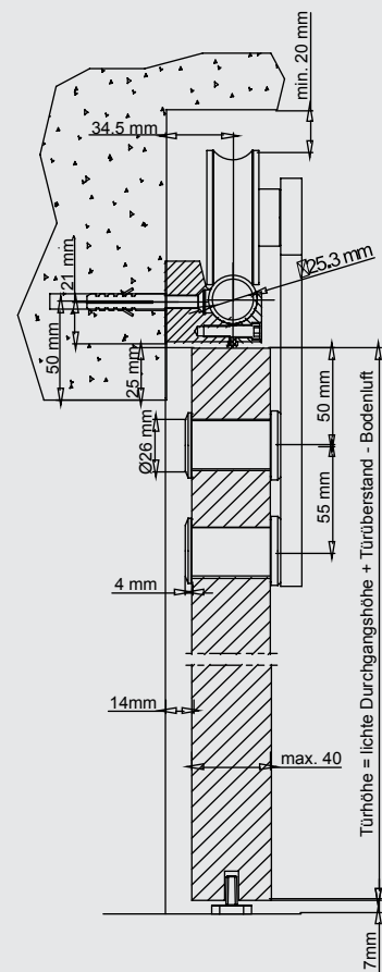
ZEICHNUNG ROTELLA PURISTO, FÜR HOLZTÜREN DRAWING ROTELLA PURISTO, FOR WOODEN-DOORS
