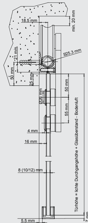
ZEICHNUNG ROTELLA PURISTO, FÜR GLASTÜREN DRAWING PURISTO, FOR GLASS-DOORS
