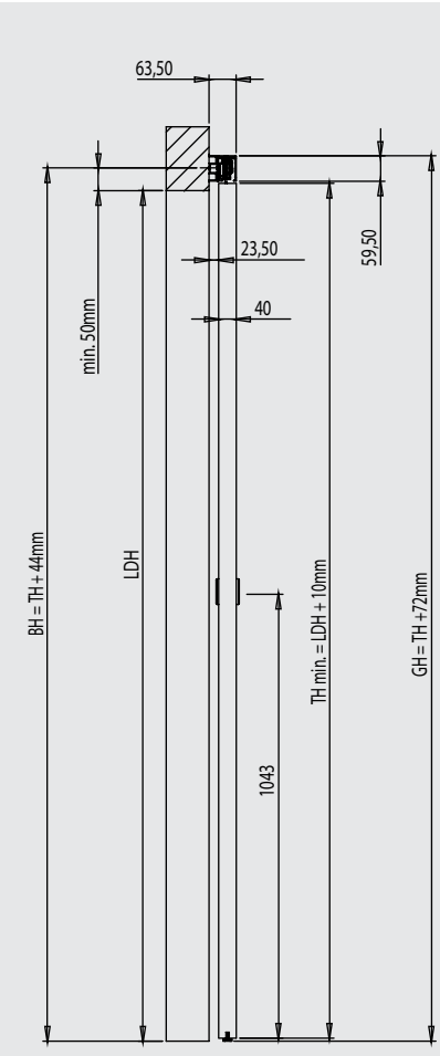
ZEICHNUNG PLANE0 50, FÜR HOLZTÜREN DRAWING PLANE0 50, FOR WOODEN-DOORS
