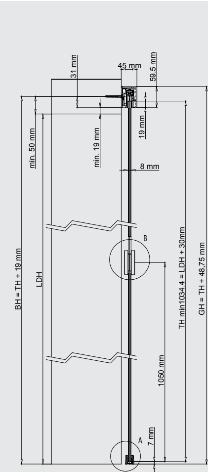
ZEICHNUNG PLANE0 50, FÜR GLASTÜREN DRAWING PLANE0 50, FOR GLASS-DOORS
